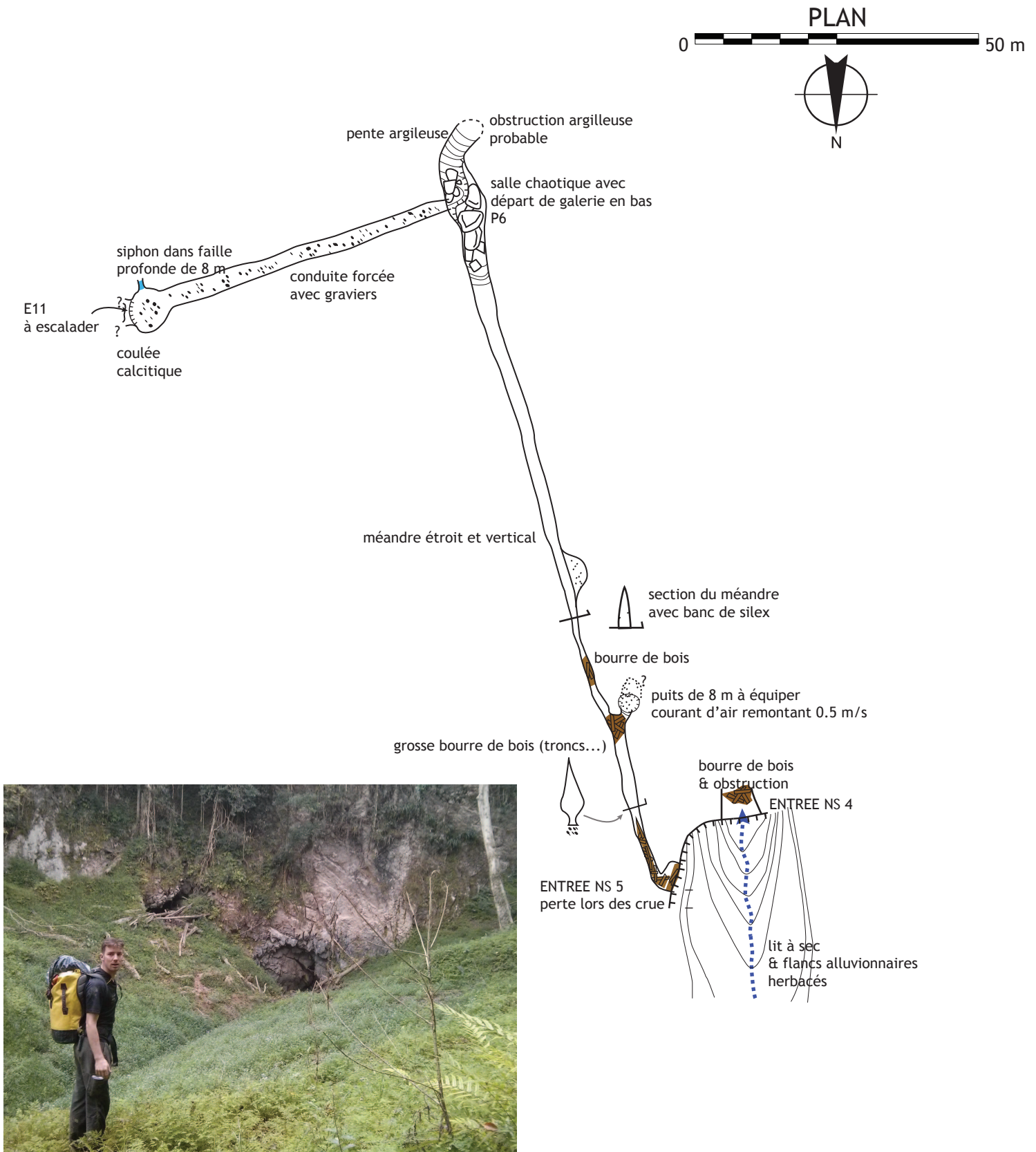
Pertes Tham Nam Sakay 5 (à gauche) et 4 (obstruée). Les dépôts alluvionnaires sont entaillés en V par le cours d'eau non-pérenne.
