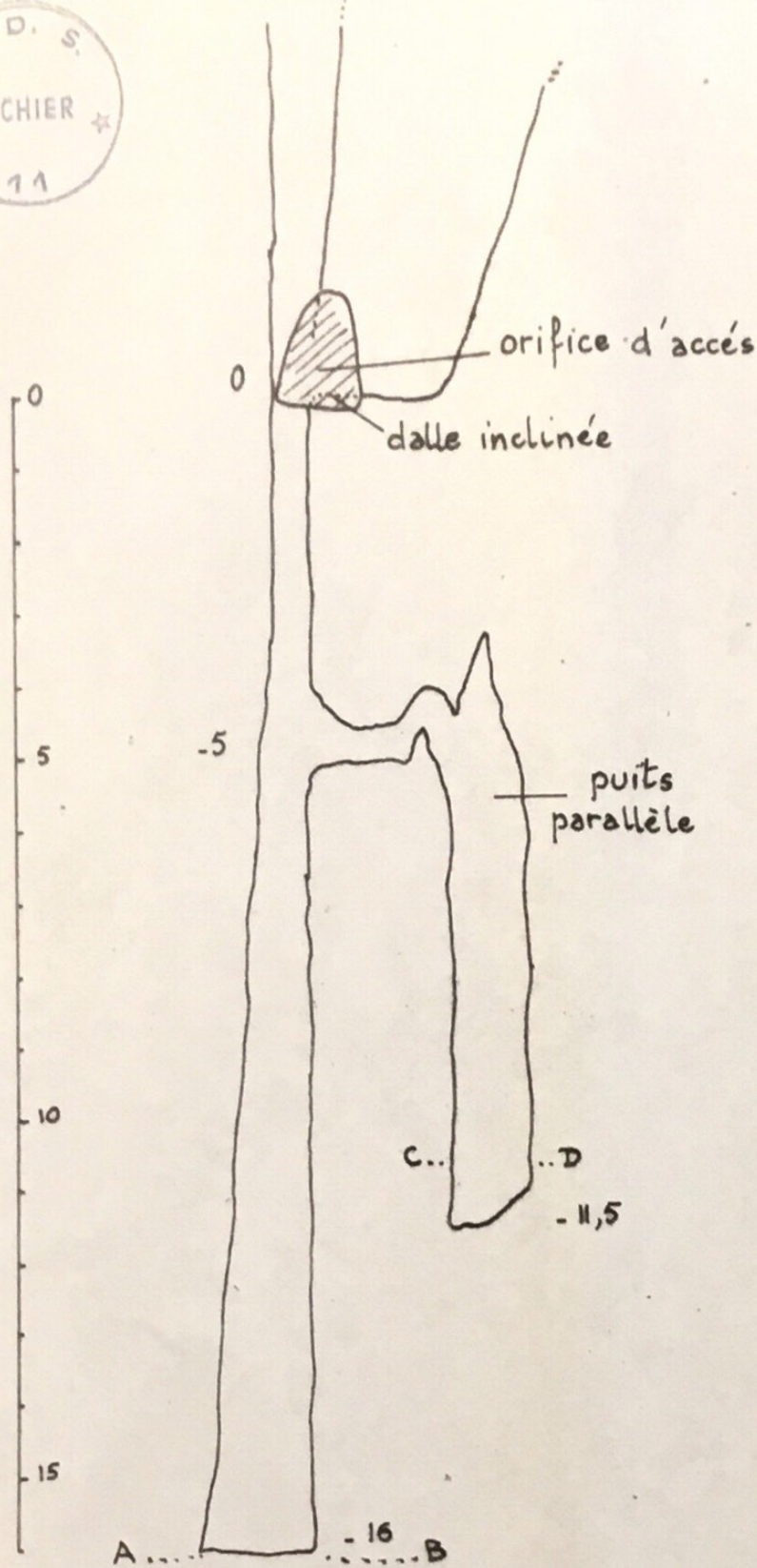
COUPE A-B
