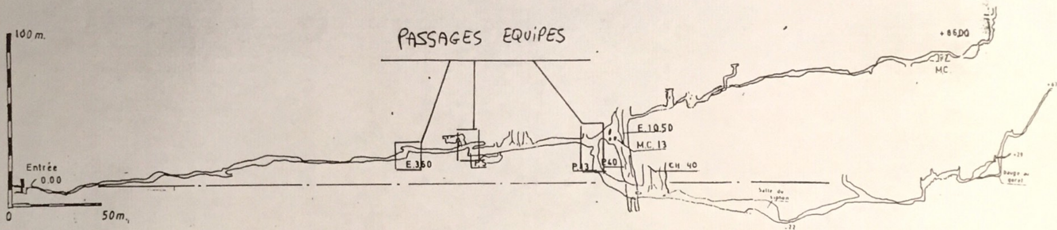
COUPE DEVELOPPEE
