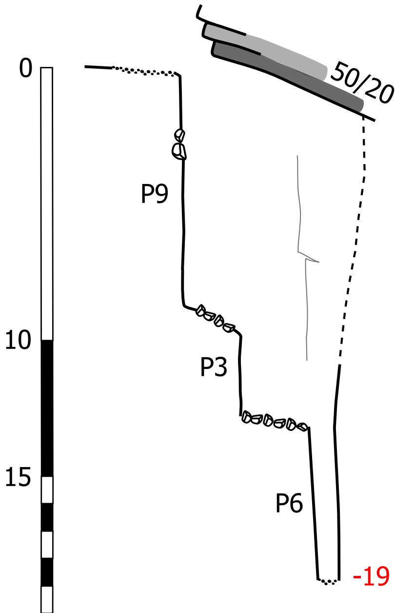
Coupe développée
